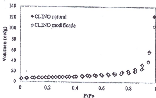
Figura 9. Isotermas de adsorción de N 2 a 77 K en zeolitas CLINO natural y CLINO modificada.
